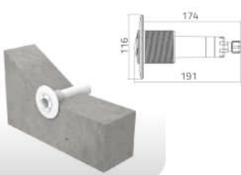
吸入管接头
