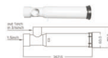
1.5" 文丘里
