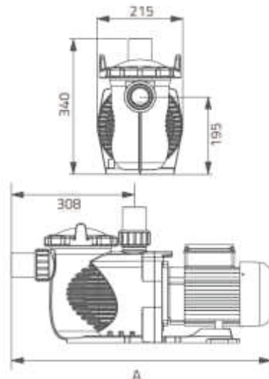
型号: SPH 水泵
