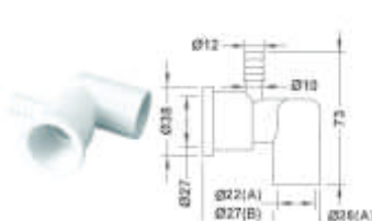
L型喷嘴身
