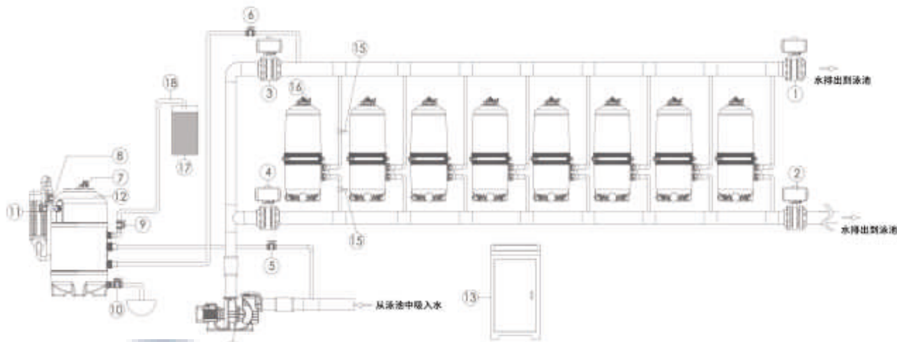
意万仕珍珠岩过滤系统由以下部分组成
