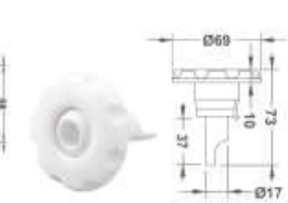
Φ2-3/4寸球型水疗喷嘴
