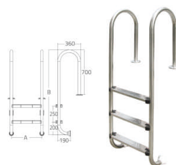
法兰不锈钢踏板
