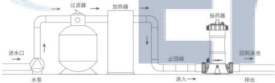
2. 型号: CL-01A/CL-02A (软管接法)
