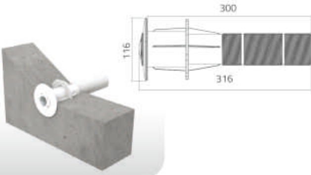
导管
