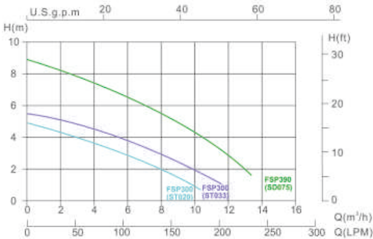
注：以上性能曲线为50Hz型号
