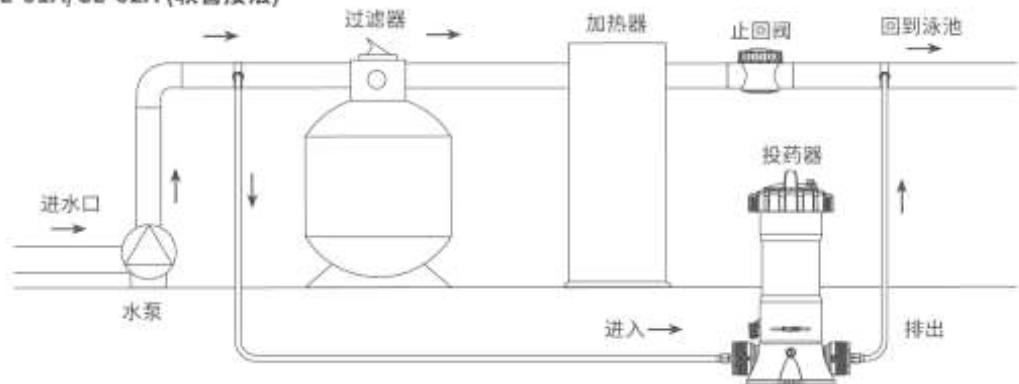
2. 型号: CL-01A/CL-02A (软管接法)
