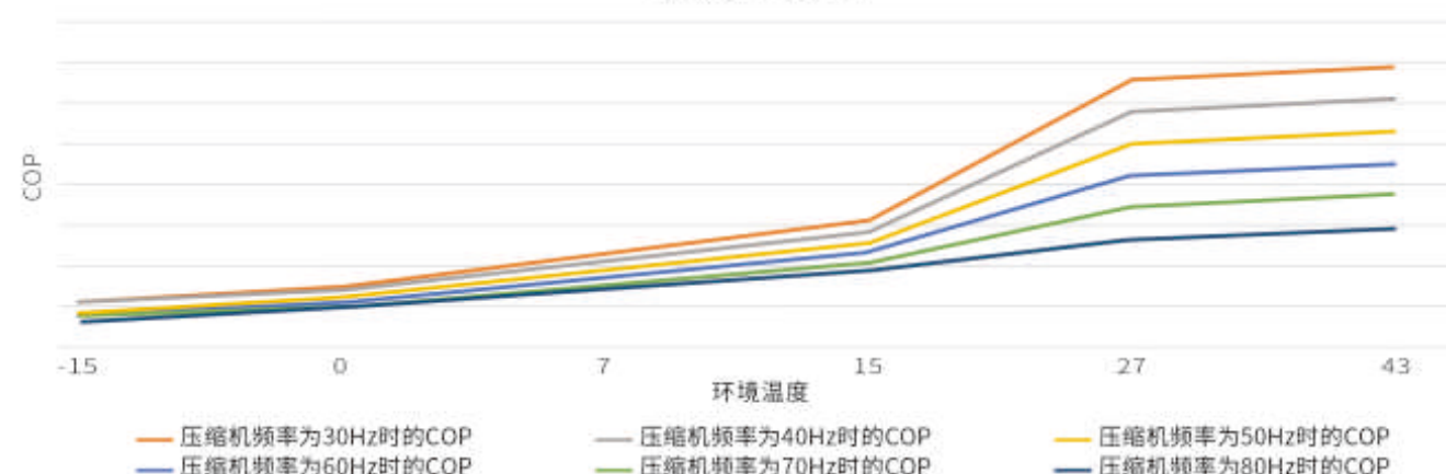
不同工况下COP的变化曲线 最大COP可达17
