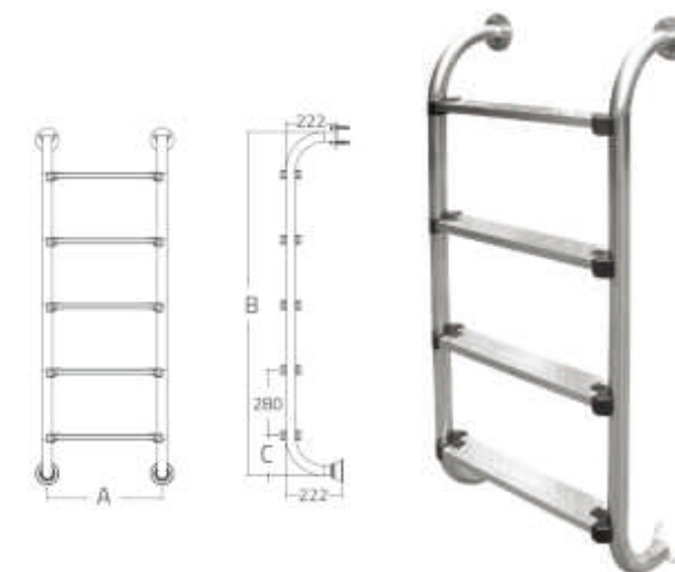
不锈钢踏板
