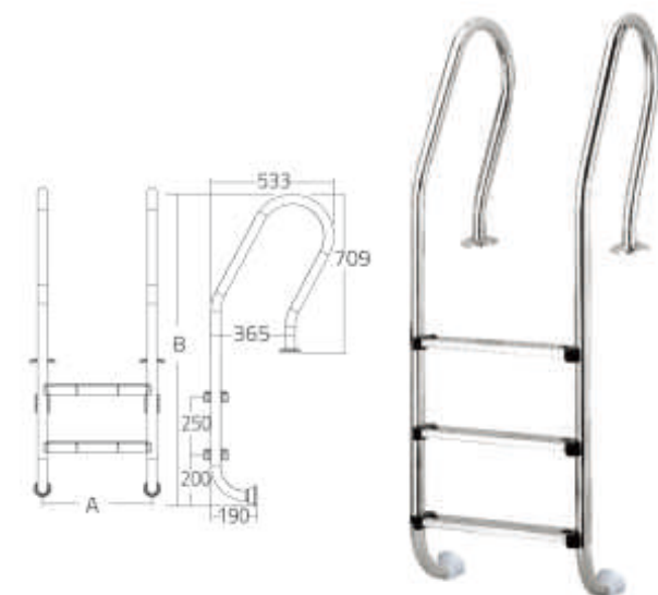
法兰不锈钢踏板
