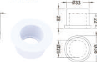
小管堵头
