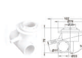
Φ10&25mm水嘴身
