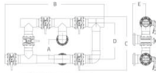
5功能蝶阀 NBV30-NBV80
